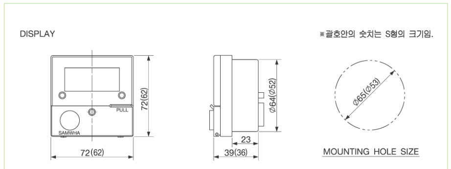
EOCR-3MZ 외부 CT 조합형 모델(100Type 이상)의 치수도
