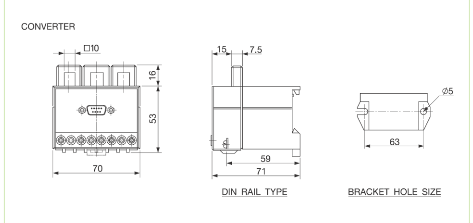
EOCR-FMZ 외부 CT 조합형 모델(100Type 이상)의 치수도
