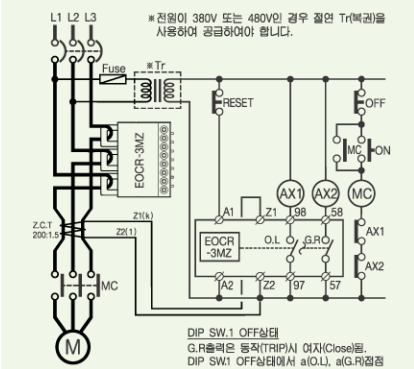
EOCR-3MZ의 Non-fail-safe형 결선 → SW1: Off설정
