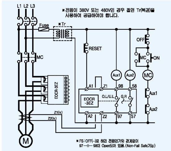
EOCR-3EZ(FS:OFF설정) 외부CT설치시
