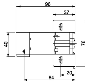
PANEL & DIN RAIL TYPE
