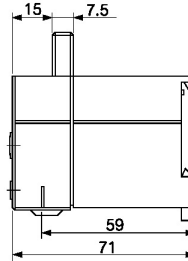
DIN RAIL TYPE
